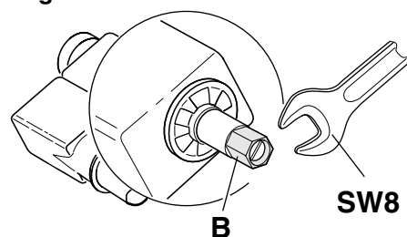
Einstellung 2. Stufe
