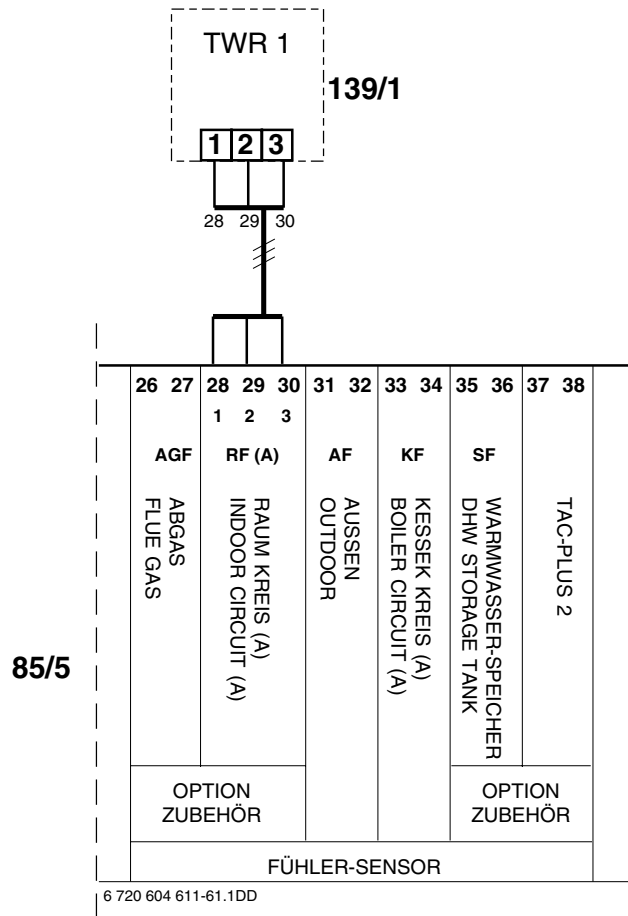
Bild 54 Anschluß ohne Zusatzleiterplatte
