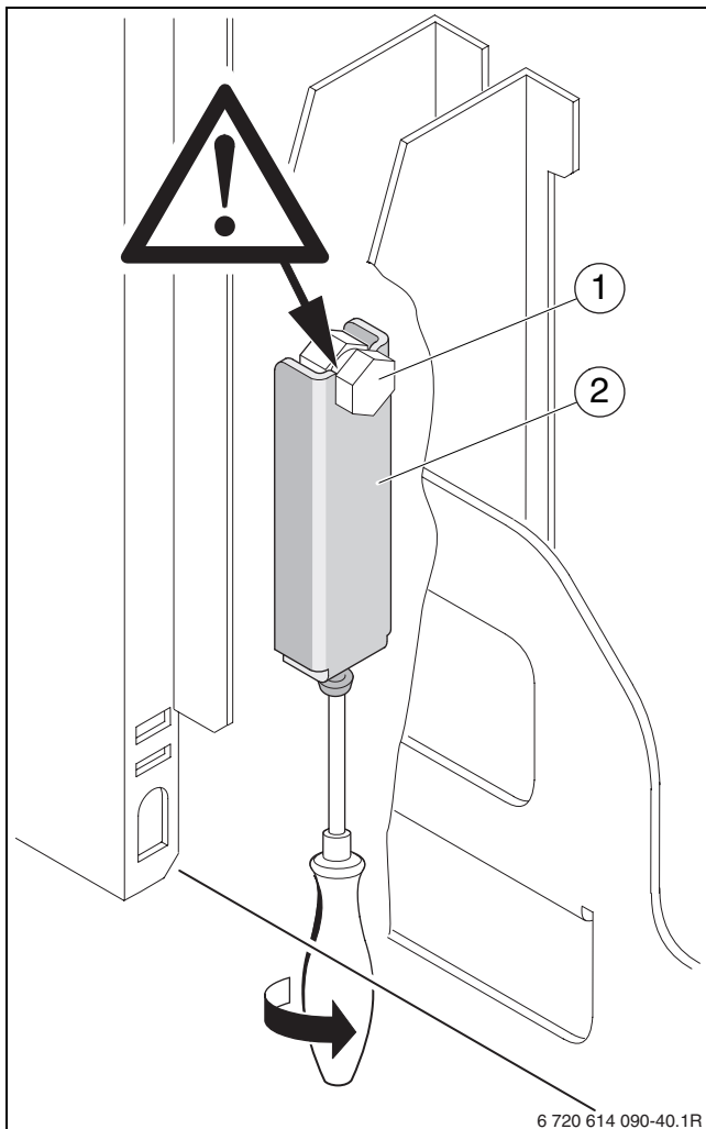
Bild 11 Verriegelung schließen
