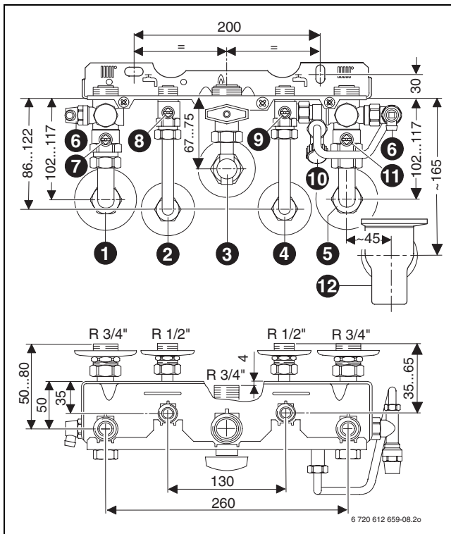
Bild 8 Beispiel: Montageanschlussplatte Nr. 1004 mit Füllinrichtung Unterputz
